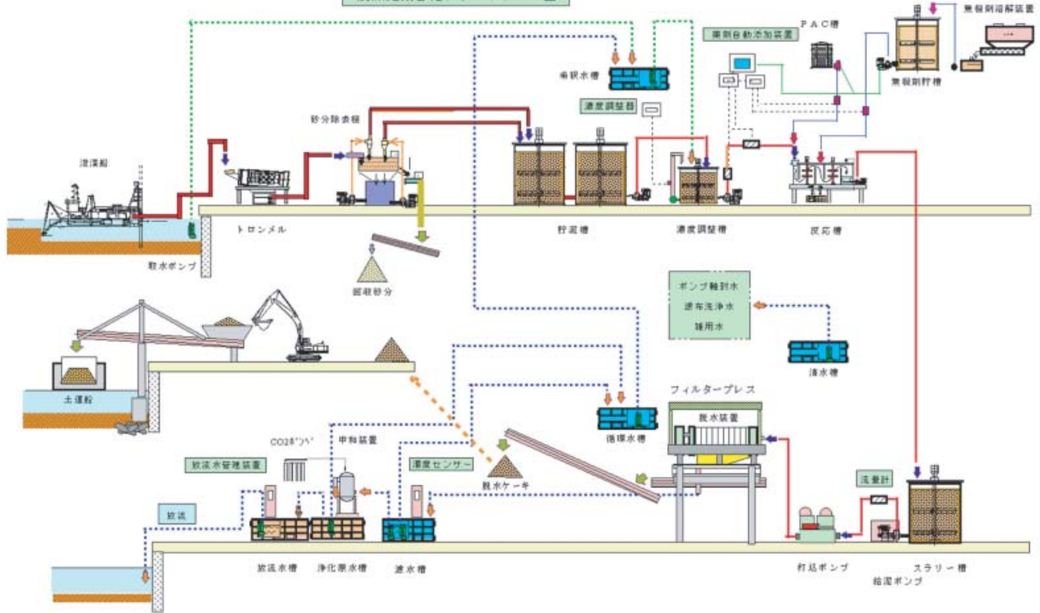
浚渫泥減容化プラントフロー図
